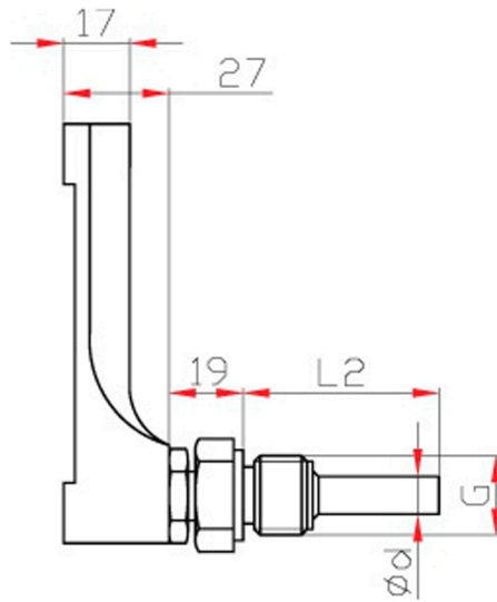
Термометры жидкостные виброустойчивые (угловое присоединение)
